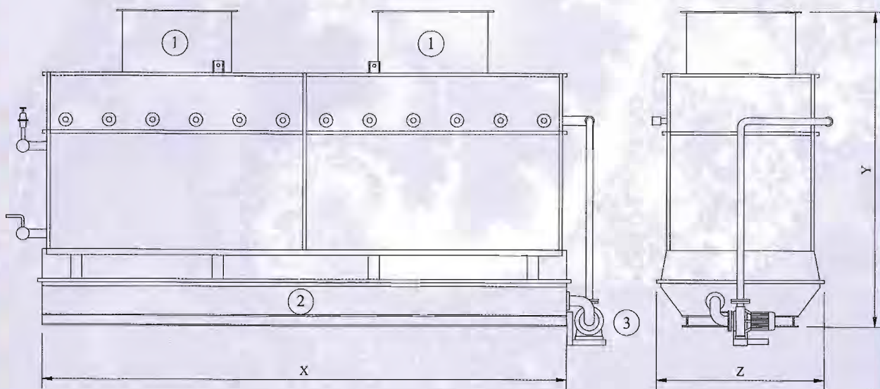
① AXIAL FAN
